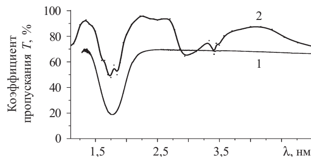
Рис. 3. Спектр пропускания активных элементов на основе монокристалла \text{ZnSe:Cr}^{2+} : 1 — непросветленный образец; 2 — просветленный образец
