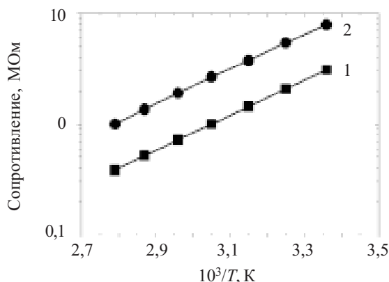
Рис. 2. Типичные эксплуатационные характеристики термомочувствительности толстых пленок оксиманганатной керамики:
