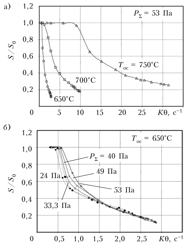
Рис. 2. Зависимость отношения S/S_0 от K\theta при осаждении пленок нелегированного ПК для различных значений T_{ос} (а) и P_{\Sigma} (б)
