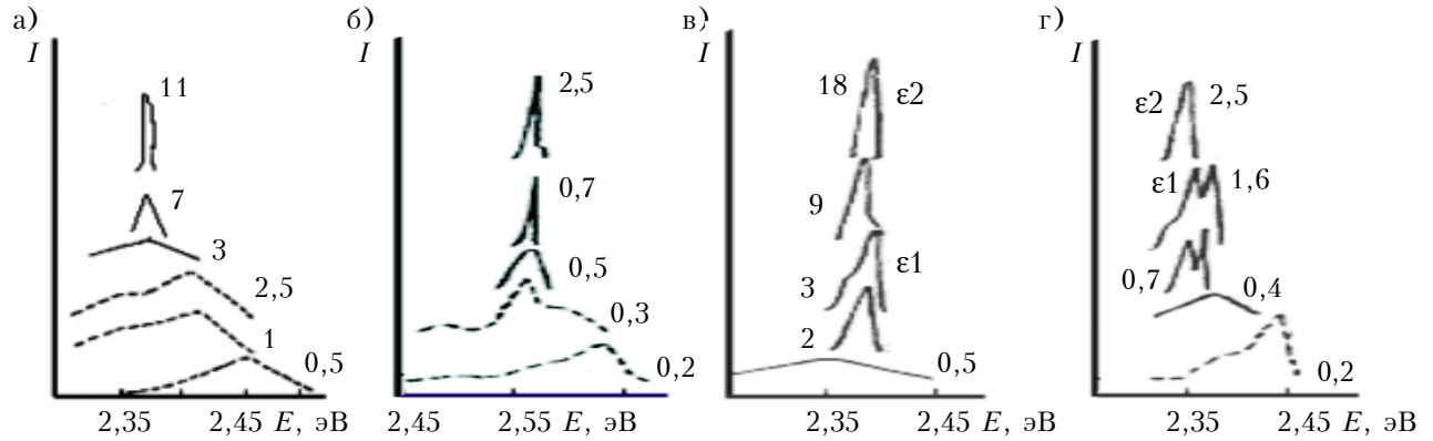
Рис. 2. Спектры катодолуминесценции (штриховые) и генерации (сплошные) кристаллов CdS, нелегированных (а, б) и радиационно легированных (в, г) изотопами Pd ( \epsilon 1 ) и Ag ( \epsilon 2 ), при 300 К (а, в) и 80 К (б, г) (Цифры возле кривых указывают плотность тока j в А/см 2 )
