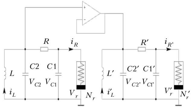
Рис. 5. Схема синхронизации генераторов Чуа сигналом V_{C2}
