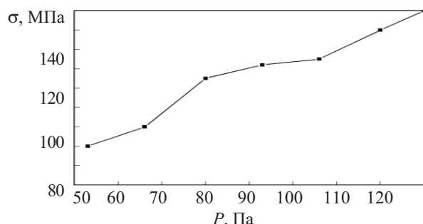
Рис. 2. Зависимость уровня внутренних механических напряжений в пленке \text{SiN}_x от давления в рабочем объеме камеры
