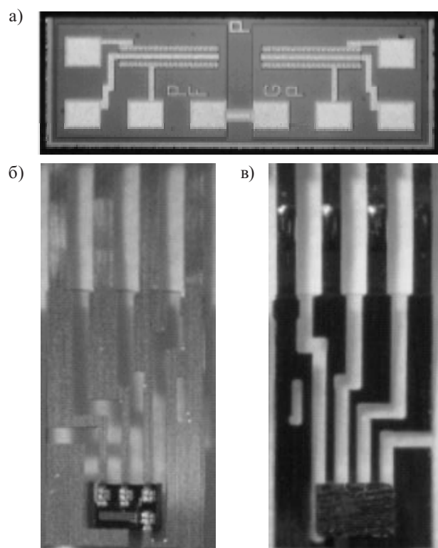
Рис. 2. Фото кристалла с прямыми p -канальными транзисторами «F» и «G» (а) и фото кристалла в сборке на гибком носителе (б — лицевая сторона, в — обратная сторона)
