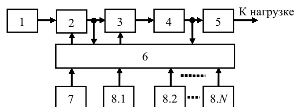
Рис. 1. Структурная схема специализированного устройства электропитания:
