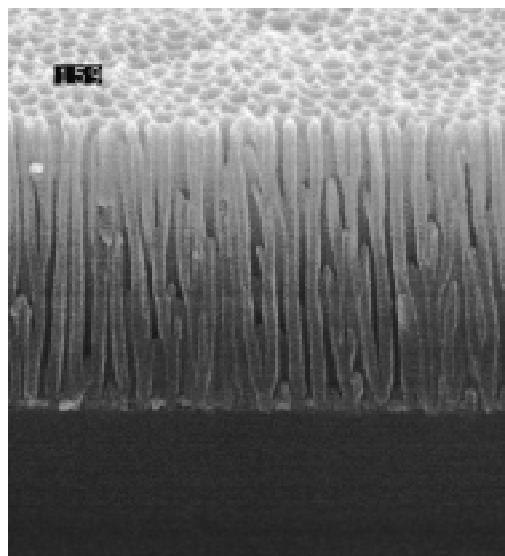
Рис. 4. Анодированный Al с растравленными порами
