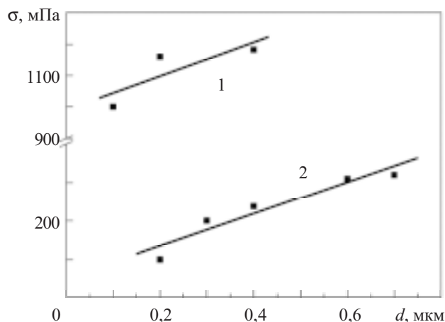
Рис. 2. Зависимость механического напряжения от толщины пленки нитрида кремния при различных отношениях объемов SiH_2Cl_2/NH_3 : 1 — 1/4; 2 — 4/1
