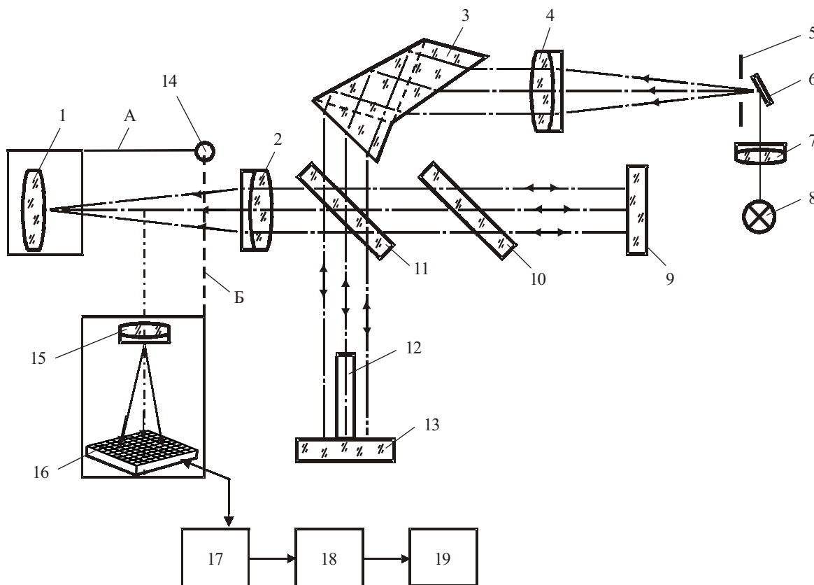
Рис. 1. Функциональная схема модернизированного интерферометра Кестерса:
