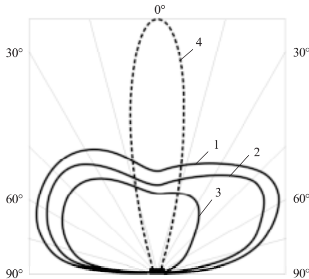
Рис. 2. ДН излучения АЭ плоской конструкции, изготовленного на основе \text{Ga}_x\text{In}_{1-x}\text{As} ( 0 \leq x \leq 0,1 ), с максимумом излучения в области 3,0—3,8 мкм: 1 — АЭ без чернения; 2 — с черненной передней гранью; 3 — с черненными передней и боковой гранями; 4 — планарный АЭ помещен в параболический отражатель
