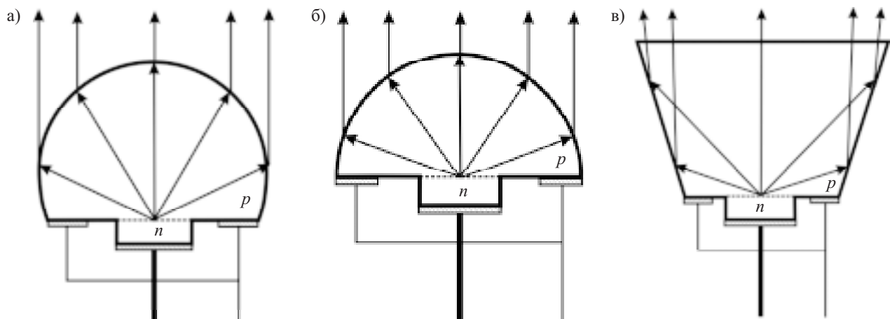
Рис. 3. Различные формы АЭ: а — сфера Веерштрасса; б — полусфера; в — усеченный конус
