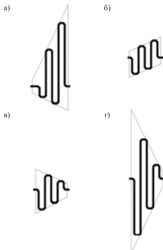
Рис. 22. Варианты направленных вниз змеек с нечетным числом полупериодов
