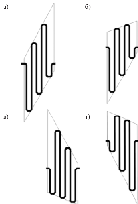
Рис. 21. Варианты направленных вниз змеек с четным числом полупериодов
