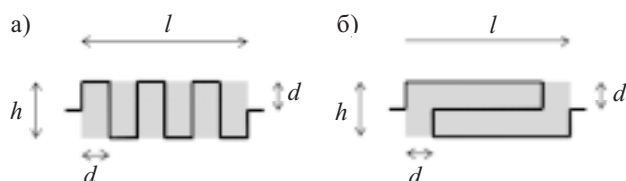
Рис. 1. Варианты вписывания меандра: а — accordion (аккордеон); б — trombone (тромбон) (по терминологии «Specetra»)
