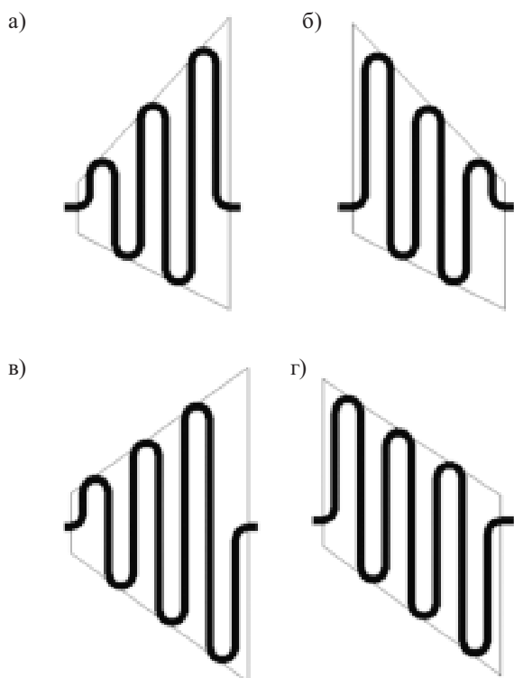
Рис. 16. Направленные вверх змейки с различными параметрами в верхнем треугольнике
