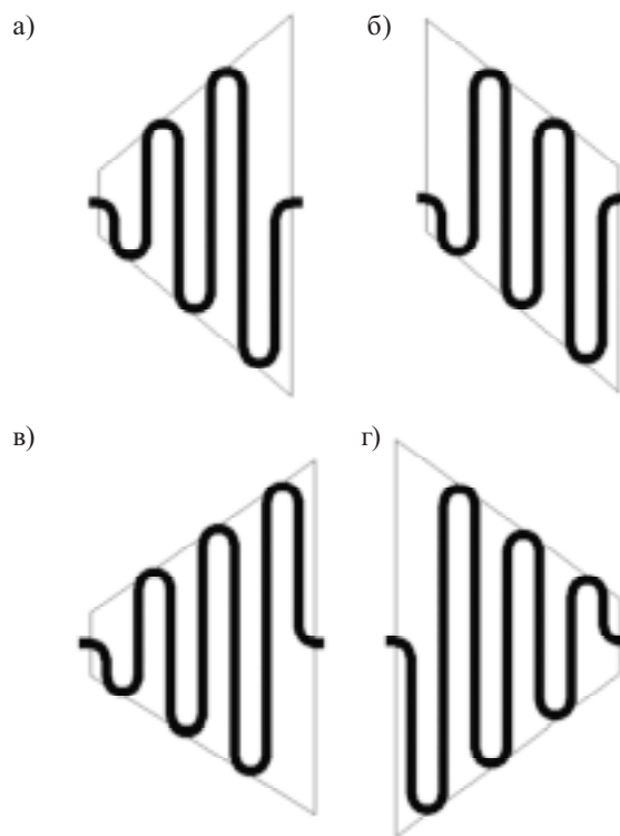
Рис. 17. Направленные вниз змейки с различными параметрами в верхнем треугольнике
