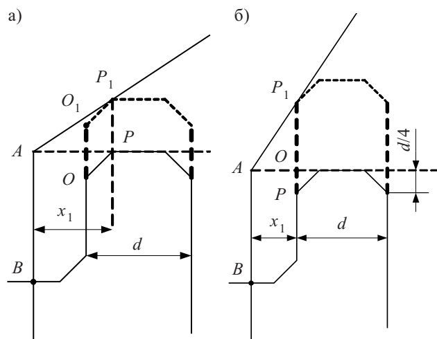
Рис. 18. Добавка длины от первого изгиба с аппроксимацией для случаев, когда угол возвышения меньше 45^\circ (а) и больше 45^\circ (б)
