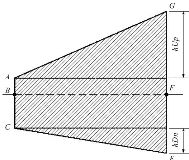
Рис. 9. Область, в которых рассчитывается длина змейки
