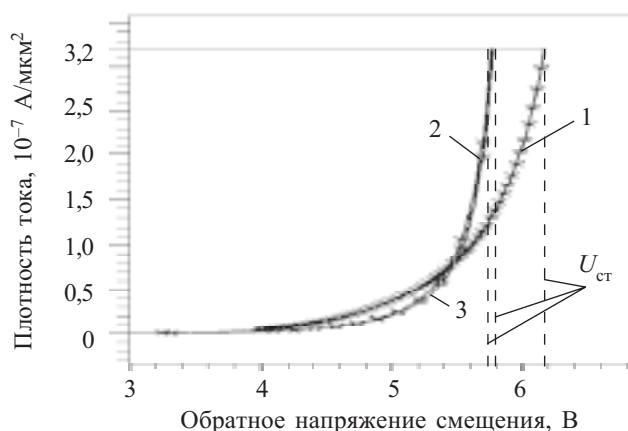
Рис. 2. Обратные ветви ВАХ стабилитрона в структурах, полученных в результате диффузионного легирования фосфором подложки типа КДБ0,003 (1); КДБ0,004 (2); КДБ0,005 (3) при комнатной температуре
