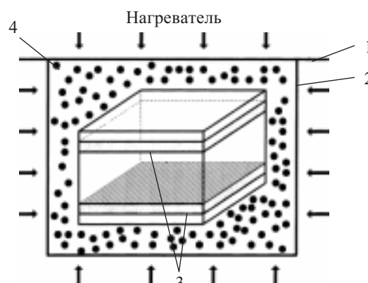
Рис. 1. Схема устройства для легирования пленок методом испарения:
