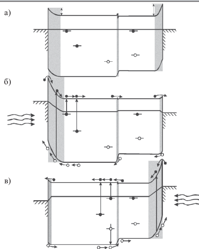
Рис. 6. Энергетическая зонная диаграмма Ag-NGaAs- n GaInAs-Ag-структуры
