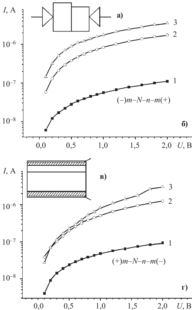
Рис. 1. BAX Ag-NGaAs-nGaInAs-Ag-структуры: 1 — в темноте; 2 — 100 лк; 3 — 1000 лк
