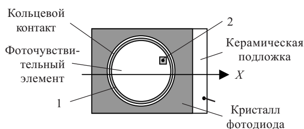
Рис. 1. Вид фотоприемника со стороны фоточувствительного элемента (X — направление сканирования ФЧЭ вдоль оси симметрии):
