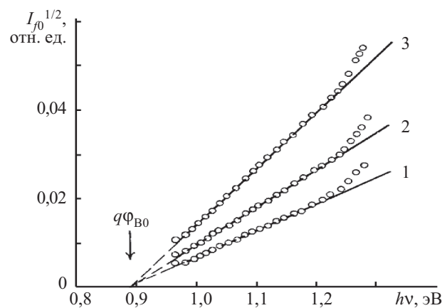
Рис. 2. Зависимость фототока от энергии фотонов для структуры Au- n -GaAs № 2 при разных направлениях освещения ( T=300 К):
