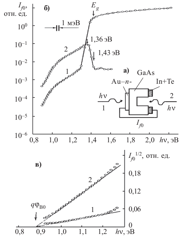
Рис. 1. Схема измерений фототока короткого замыкания I_{f0} в структурах Au- n -GaAs (а) и зависимости фототока ( I_{f0} , I_{f0}^{1/2} ) от энергии фотона ( h\nu ) для структуры № 1 (б, в): 1 — освещение со стороны Au; 2 — освещение со стороны GaAs (T=300 K)
