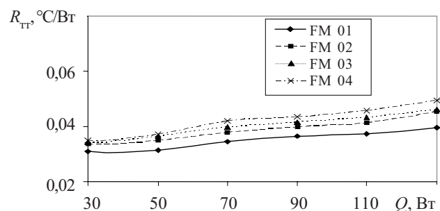
Рис. 7. Зависимость термического сопротивления ТТ от величины передаваемого теплового потока при t_v=30^\circ\text{C}
