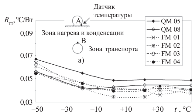
Рис. 6. Зависимость термического сопротивления ТТ от температуры пара при Q=90 Вт и схема расположения термопар (а)
