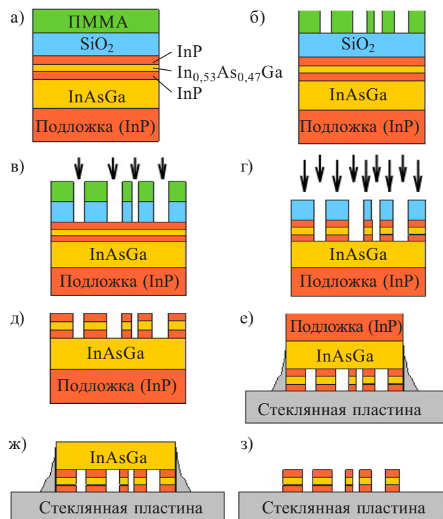
Рис. 1. Процесс изготовления двумерных ФК на полупроводниковых подложках:
