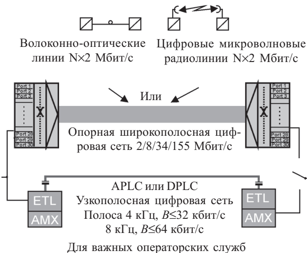
Рис. 5. Обобщенное построение корпоративной сети связи энергетических предприятий
