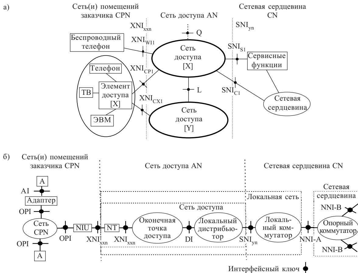
Рис. 3. Эталонная модель транспорта сети доступа ANT RM: а — логическое представление; б — физическое представление
