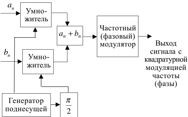
Рис. 1. Структурная схема модулятора с квадратурным изменением угловой компоненты
