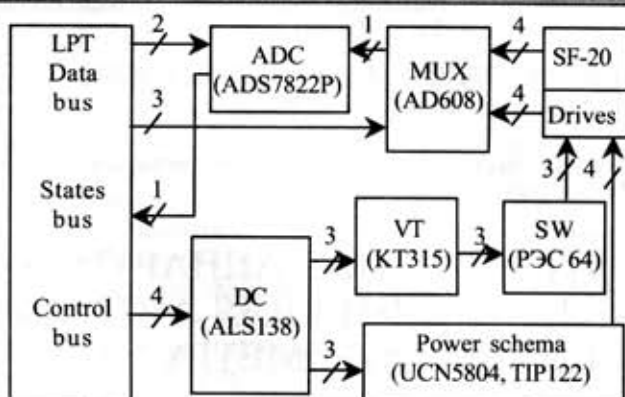
Рис. 1. Функциональная схема устройства сопряжения спектрофотометра СФ-20 с компьютером
