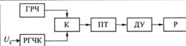
Рис. 4. Структурная схема пьезоэлектрического ионизатора воздуха с плавной регулировкой производительности
