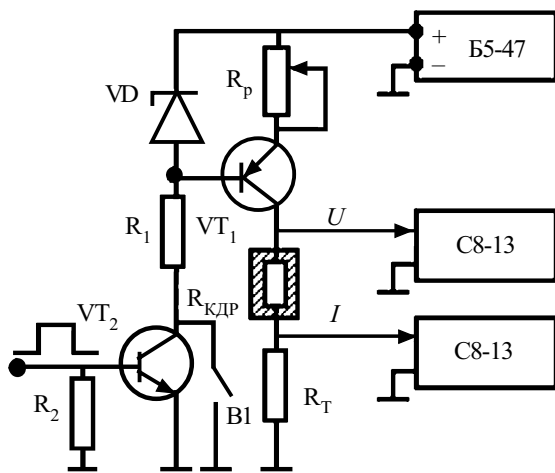
Рис. 2. Схема измерений
