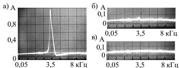
Рис. 2. Амплитудно-частотные характеристики пьезопреобразователей:
