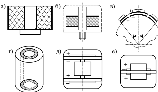
Рис. 8. Конструкции акселерометров
