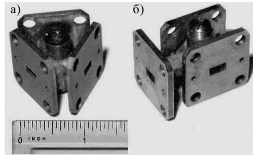
Рис. 4. Волноводные Y-циркулятор (а) и Т-циркулятор (б) КВЧ-диапазона длин волн
