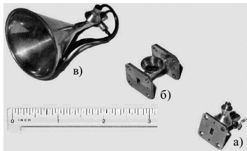
Рис. 2. Элементы и узлы КВЧ-диапазона: а — генератор на диоде Ганна со стабилизирующим биконическим резонатором; б — биконический резонатор в разобранном виде; в — автодинный преобразователь частоты на диоде Ганна с рупорной антенной
