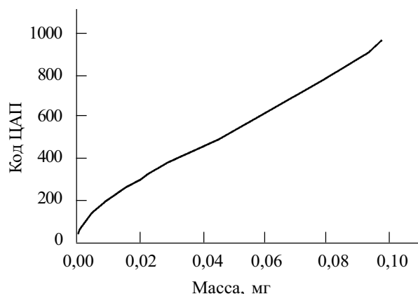
Рис. 4. Калибровочный график
