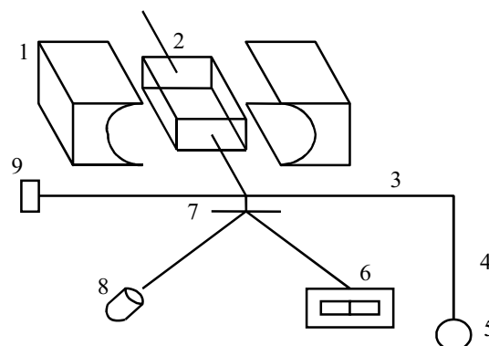
Рис. 1. Структурная схема преобразователя
