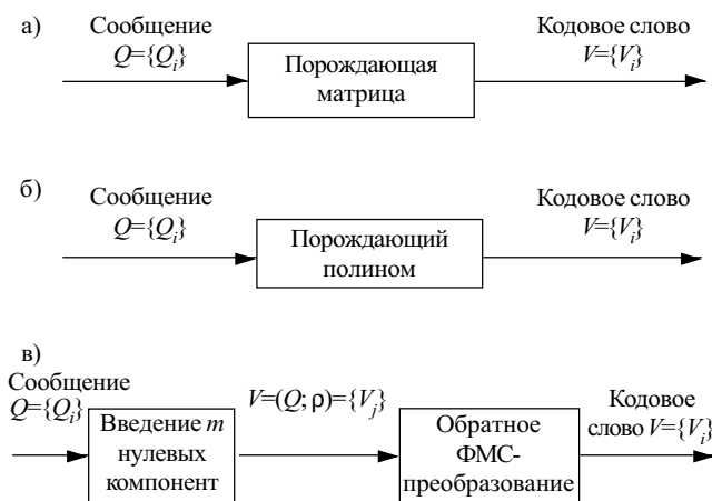
Рис. 3. Обобщенные структуры кодеров РС-кодеров: во временной области — линейного (а) и циклического (б); в частотной области — в; i=1, 2, \dots, k; j=1, 2, \dots, n=k+m; p=(0\dots 0)t нулей
