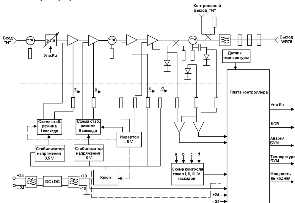
Рис. 2. Структурная схема БУМ 5
