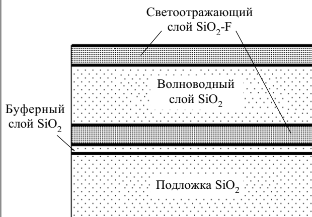
Рис. 5. Поперечное сечение волноводной структуры на основе \text{SiO}_2
