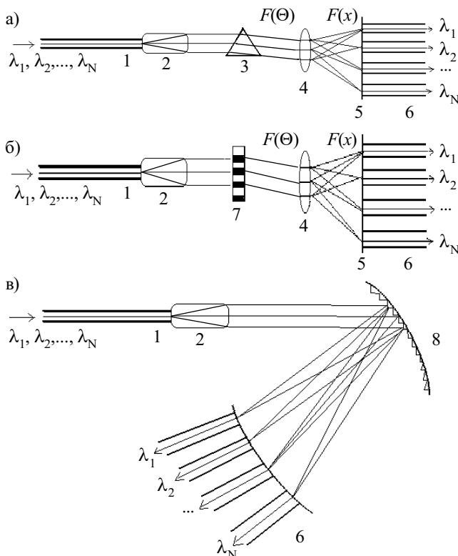
Рис. 2. Схемы основных типов объемных демультиплексоров на основе призмы (а), дифракционной решетки проходящего типа (б), на основе отражательной дифракционной решетки (в):
