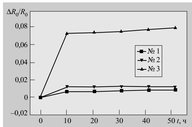
Рис. 3. Долгосрочная стабильность при температуре таяния льда
