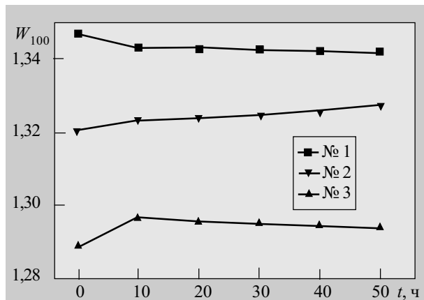
Рис. 4. Долгосрочная стабильность W_{100}
