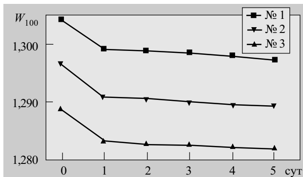
Рис. 2. Кратковременная стабильность W_{100}
