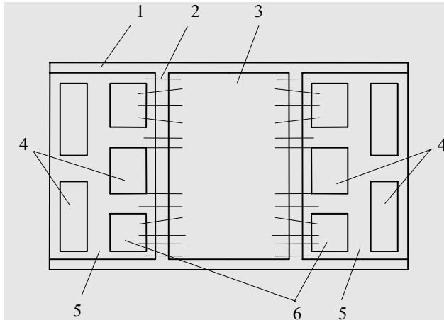
1 — основание; 2 — межплатные перемычки; 3 — тонкопленочная плата; 4 — реактивные компоненты; 5 — однослойная печатная плата; 6 — полупроводниковые приборы
