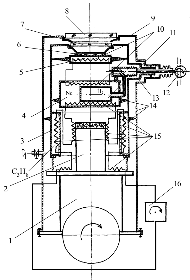
Рис. 4. ФПУ на основе ГKM Стирлинга с аккумуляторами холода на твердом неоне:
