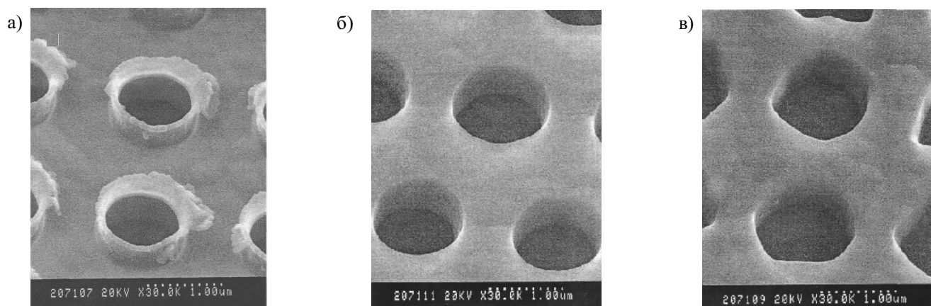
Рис. 3. Фотографии контактов-2:
