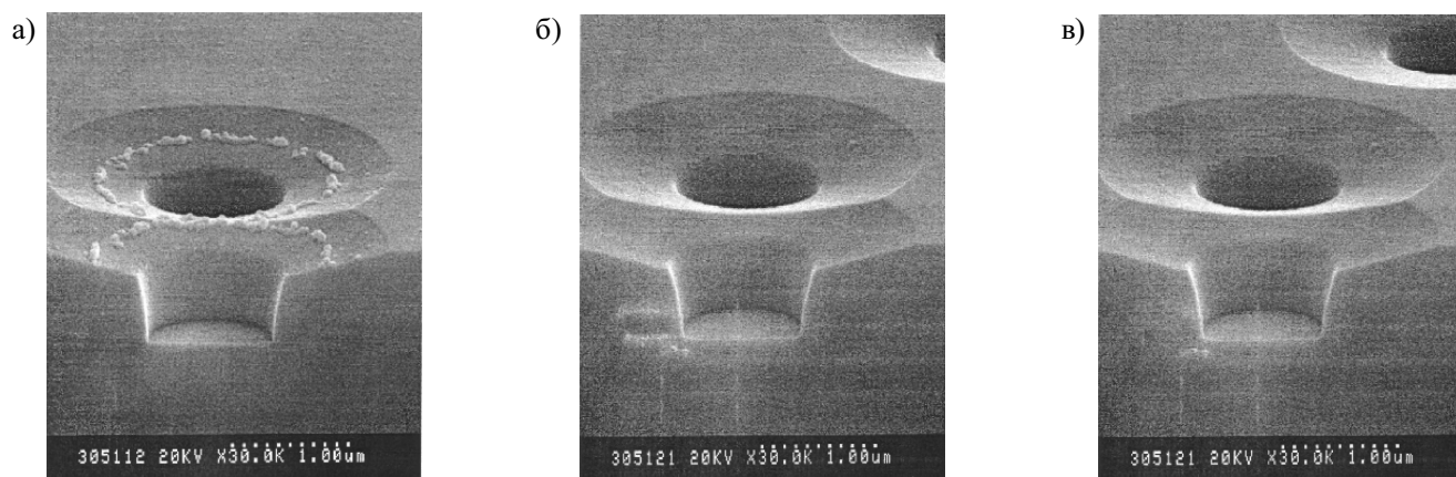
Рис. 2. Фотографии контактов-1:
