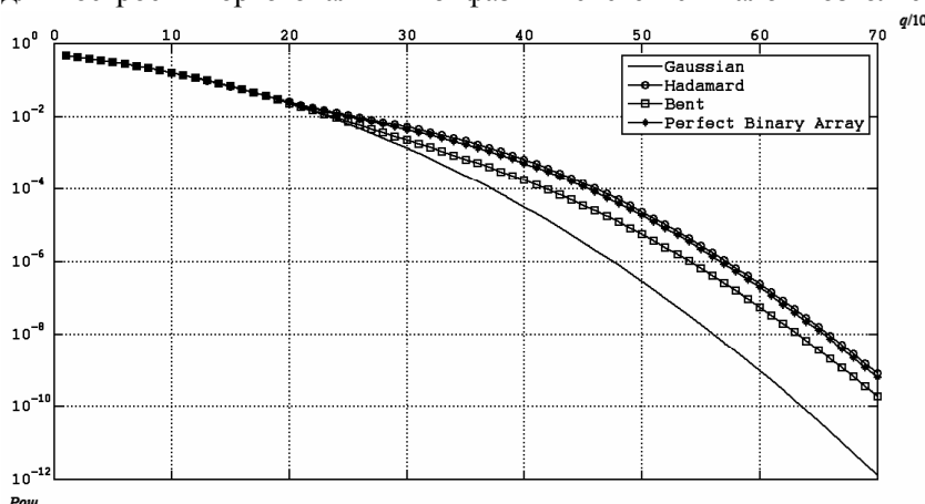
График зависимости вероятности ошибки от отношения сигнал/взаимная помеха
