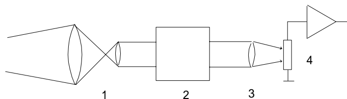
Структурная схема приемного устройства тепловизионной системы:
