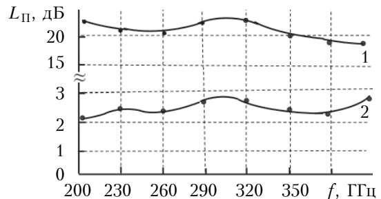
Рис. 15. Частотные зависимости потерь пропускания (1) и потерь запирающего (2) решетчатой поверхности ориентированных p-i-n -структур
