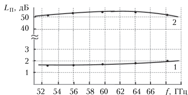
Рис. 6. Частотные характеристики потерь пропускания (1) и потерь запирания (2) выключателя, представленного на рис. 4
