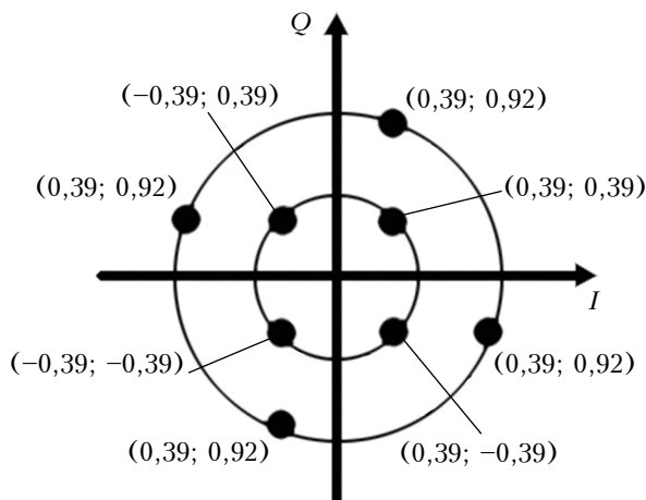
Рис. 3. Сузір'я сигналу з модуляцією 8-QAM
