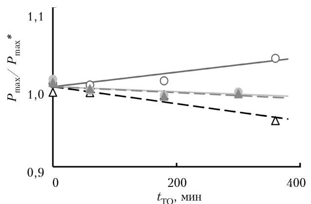
Рис. 6. Зависимость максимальной мощности, отдаваемой ФЭП, от длительности термообработки t_{TO} , проведенной при температуре 150°C для различных режимов освещения и состояний выводов (обозначения такие же, как и на рис. 2)
