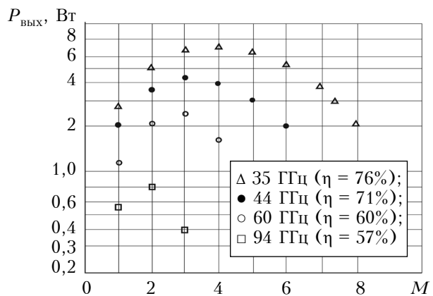
Рис. 4. Расчетные зависимости выходной мощности ISIS-диода в непрерывном режиме от количества p – n -переходов для различных значений частоты при температуре полупроводниковой структуры 140^\circ\text{C} [11]
