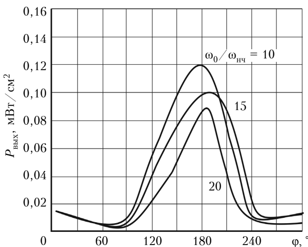
Рис. 9. Зависимость выходной мощности P_{\text{вых}} в нагрузке ВЧ-контура от фазы \varphi напряжения НЧ-сигнала при различных значениях его частоты
