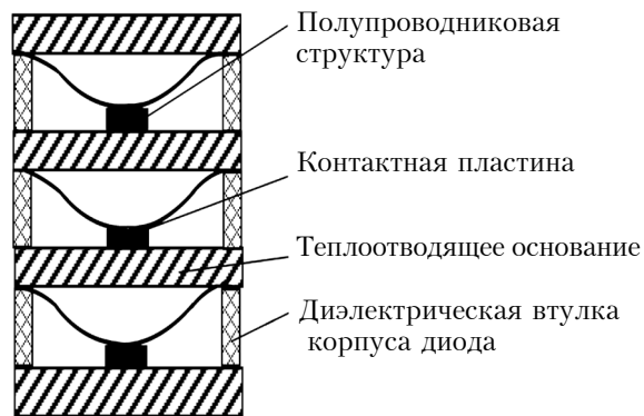
Рис. 2. Составной варакторный умножитель [9]
