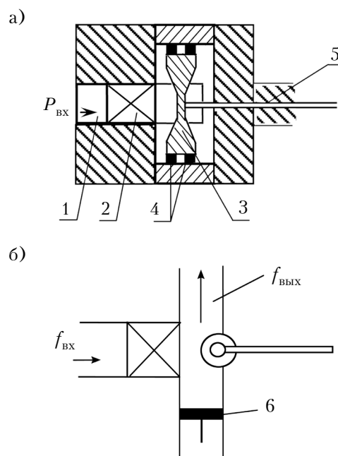
Рис. 7. Конструкция (а) и схема (б) импульсного умножителя частоты [14]
