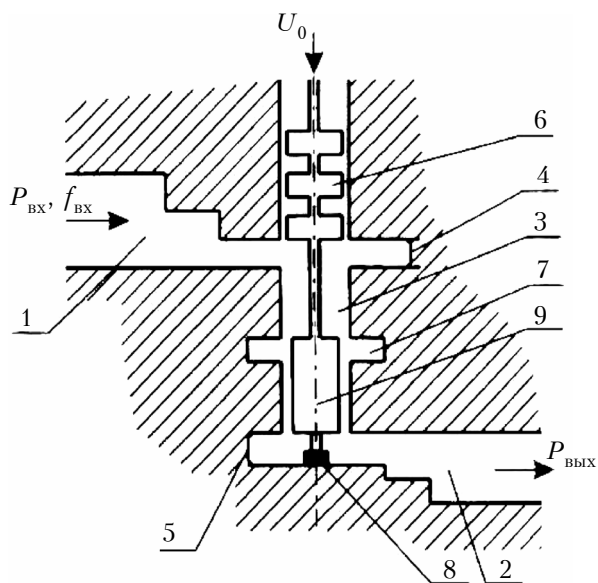
Рис. 5. Схема волноводно-коаксиальной конструкции умножителя частоты с двухслойным ISIS-диодом [12]
