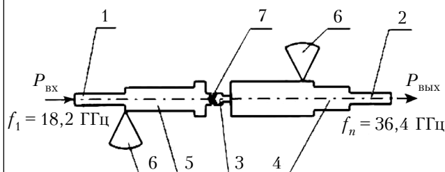
Рис. 6. Схема удвоителя частоты волн 8-мм диапазона в монокристаллическом или гибридно-интегральном исполнении с ISIS-диодом [13]
