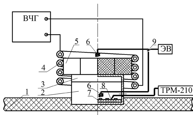
Рис. 5. Схема ВЧ-нагрева для герметизации корпусов микроблоков:
