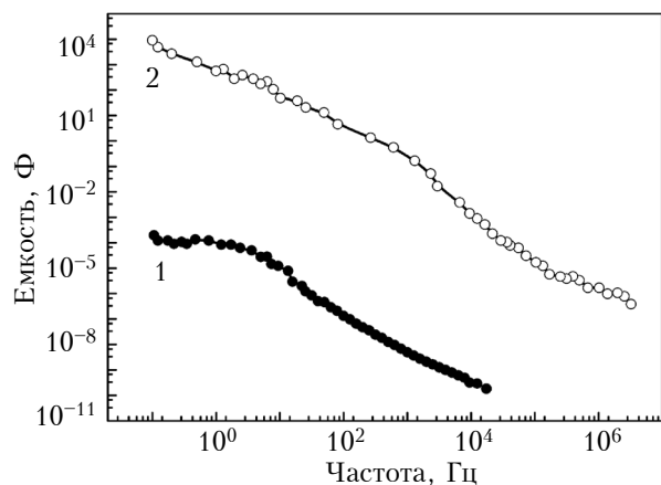
Рис. 4. Частотная зависимость электрической емкости фотоконденсатора на основе \text{InSe}\langle\text{RbNO}_3\rangle при U_{\text{см}} = 8 В в темноте (1) и при освещении (2)
