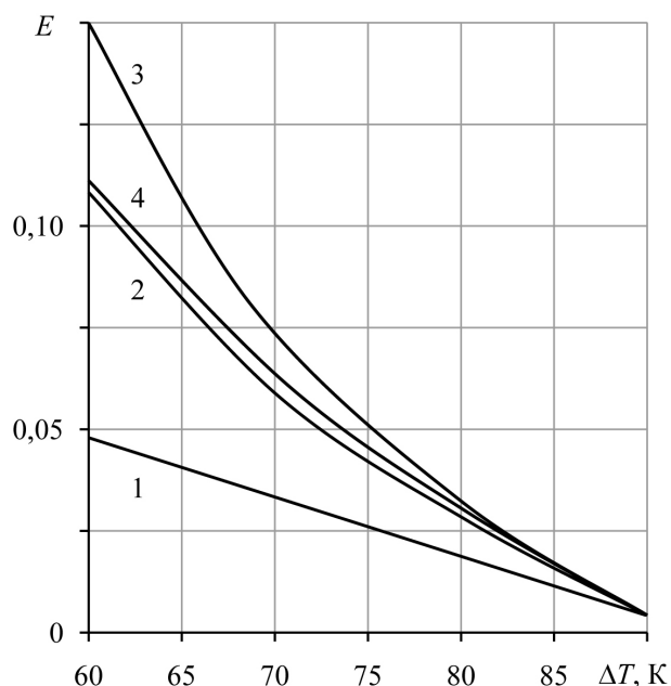
Рис. 5. Зависимость холодильного коэффициента E двухкаскадного ТЭУ от общего перепада температуры \Delta T для различных режимов работы и конфигурации ветвей термоэлементов при T = 300 К; Q_0 = 2 Вт: 1 — Q_{0\max} ; 2 — (Q_0/I)_{\max} ; 3 — (Q_0/I^2)_{\max} ; 4 — \lambda_{\min}
