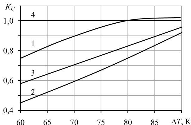
Рис. 10. Зависимость критерия K_{\Sigma} от общего перепада температуры \Delta T при T = 300 К; Q_0 = 2 Вт:
