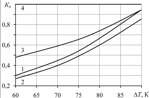
Рис. 8. Зависимость критерия K_n от общего перепада температуры \Delta T при T = 300 К; Q_0 = 2 Вт:
