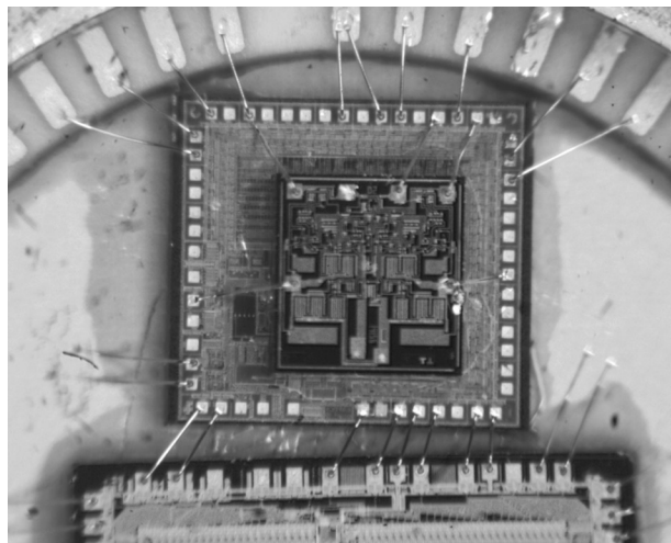
Рис. 5. Многокристаллический модуль в металлокерамическом корпусе с проволочными межсоединениями типа «шарик — клин»
