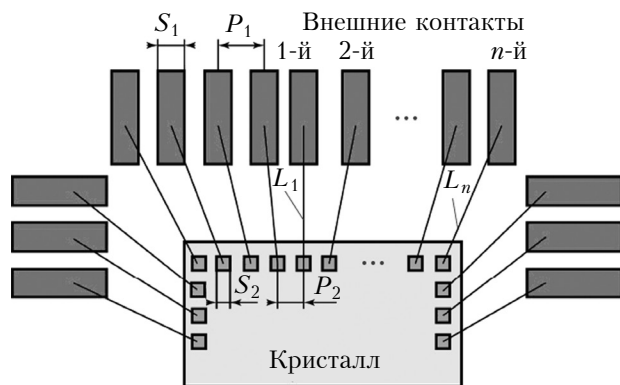
Рис. 2. Схема проволочных межсоединений между контактными площадками кристалла и корпуса прибора
