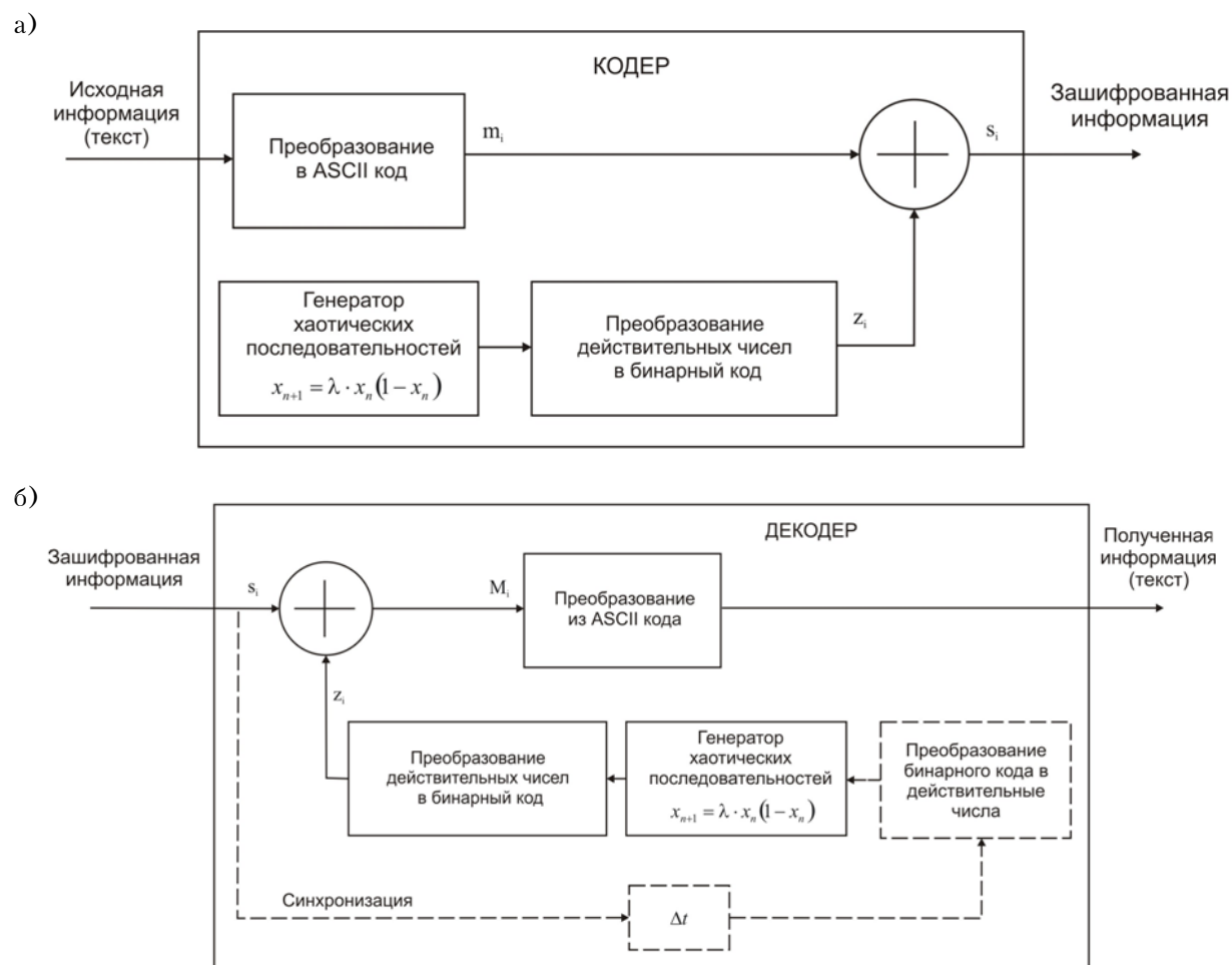
Рис. 2. Структурные схемы кодера (а) и декодера (б) системы передачи информации
