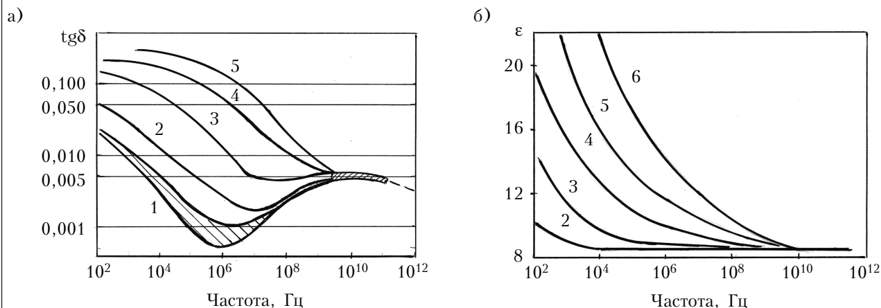
Рис. 1. Зависимость диэлектрических характеристик \text{tg}\delta (а) и \epsilon (б) от частоты в AlN-керамике при разной температуре ( ^{\circ}\text{C} ): 1 – 20–50; 2 – 100; 3 – 200; 4 – 300; 5 – 400; 6 – 500
